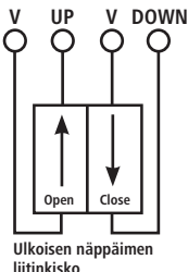
Ulkaisen näppäimen liittinkisko
