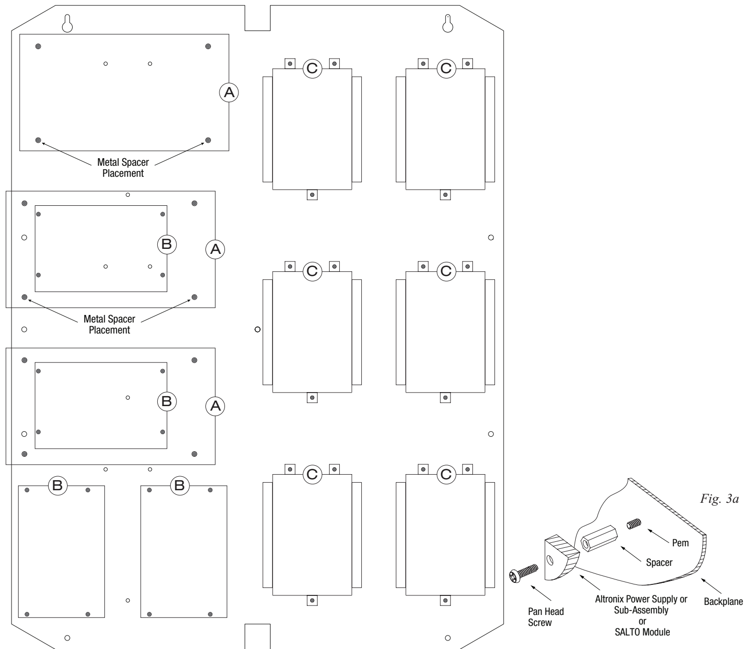
Fig. 3 - Trove2SA2/TSA2 Altronix/SALTO Configuration
