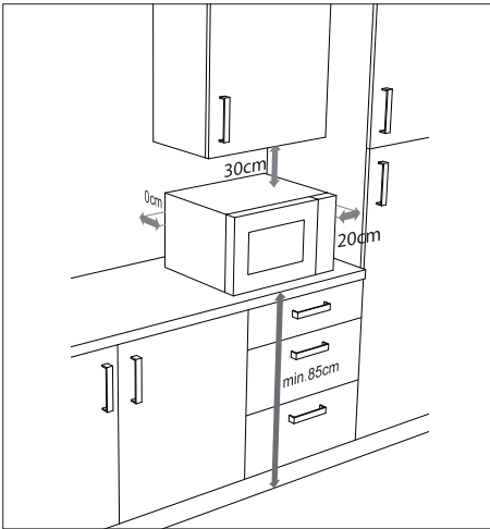
Abb. 4 – Geräteabstand
