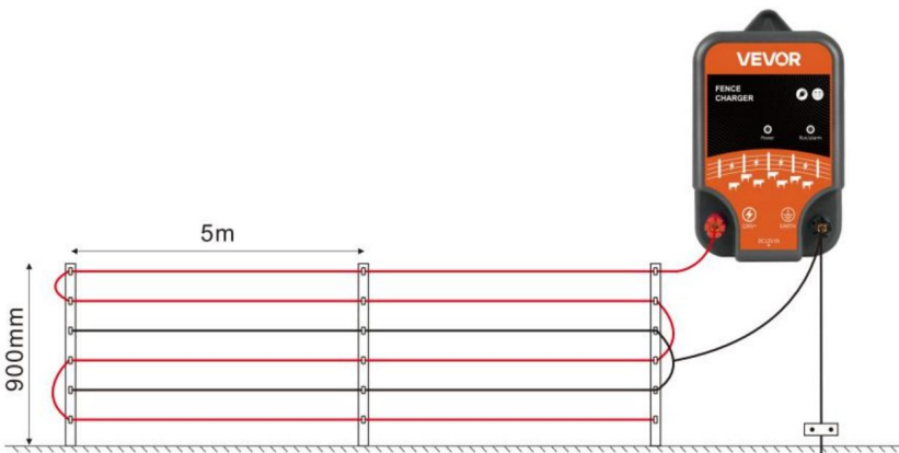
Sechs-Draht-Schaltplan
