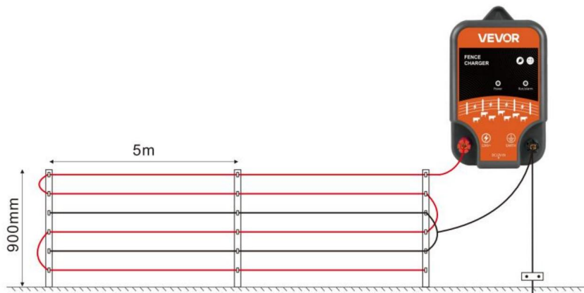
Schemat okablowania sześćożyłowego
