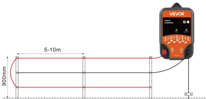
Schéma de câblage à trois fils
