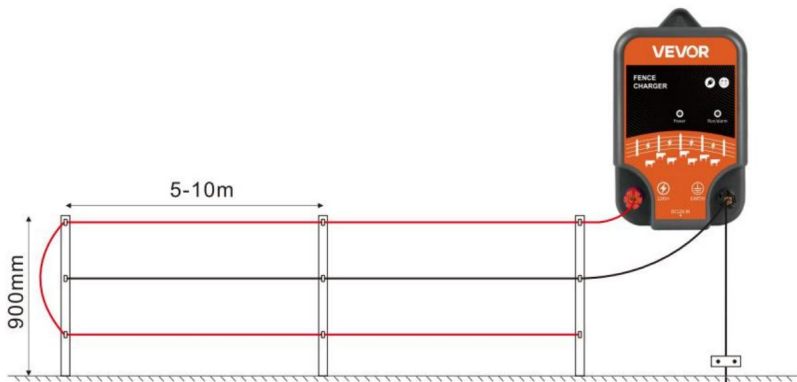
Schema voor bedrading met drie draden
