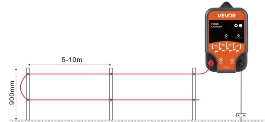
Schema voor bedrading met twee draden
