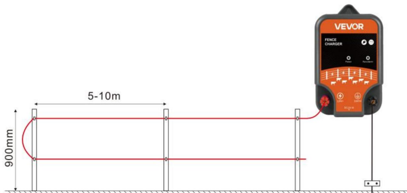
Schemat okablowania dwuprzewodowego
