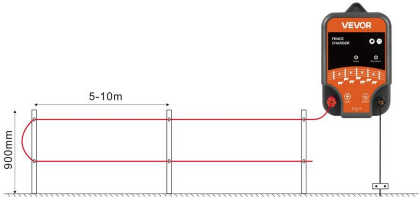
Schéma de câblage à deux fils
