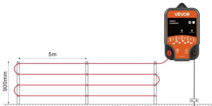
Vierleiter-Schaltplan
