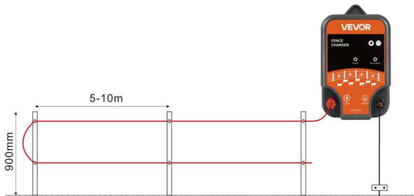
Schema elettrico a due fili
