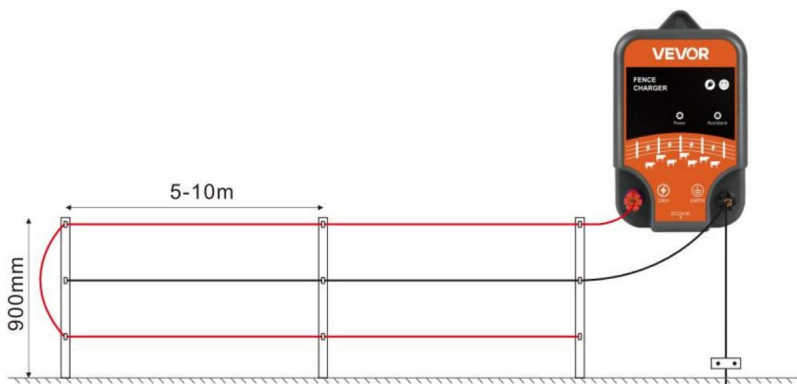
Schema elettrico a tre fili
