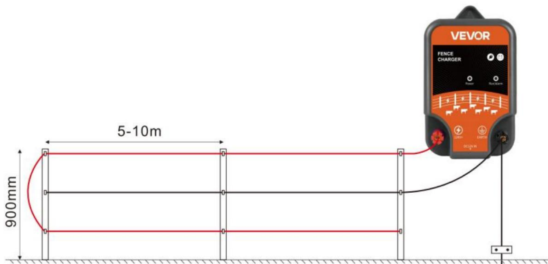
Dreileiter-Schaltplan
