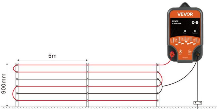
Sextråds kopplingsschema
