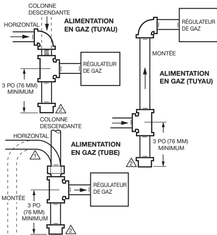
△ TOUS LES COUDES DES TUBES MÉTALLIQUES DOIVENT ÊTRE LISSES. △ MISE EN GARDE: COUPER L'ARRIVÉE DE GAZ PRINCIPALE AVANT DE RETIRER LE CAPUCHON D'EXTREMITÉ POUR EMPÊCHER QUE LE GAZ NE REMPLISSE LA ZONE DE TRAVAIL. EFFECTUER UN TEST DE FUITE DE GAZ UNE FOIS L'INSTALLATION TERMINÉE.
