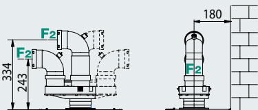
Model FF - Ayrık veya yalnızca pis hava atış baca çıkışı
