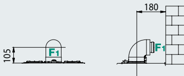
Model FF - İç içe (koaksiyal) baca çıkışı
