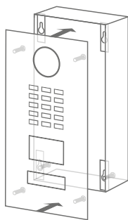
1.) Frontblende in das Montagerückgehäuse drücken.
