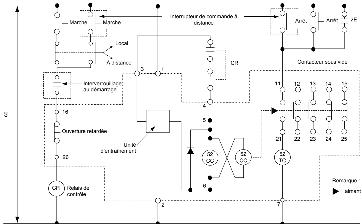
Figure 7 : Schéma de circuit de fonctionnement standard pour un contacteur à accrochage mécanique utilisant un déclencheur shunt
