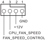
CPU_FAN1
