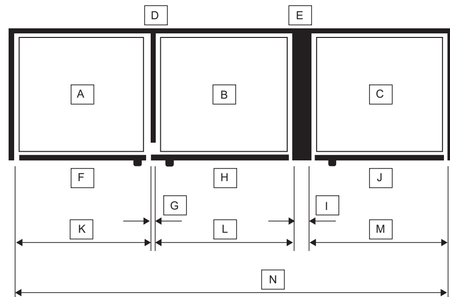
Schéma D – Toutes les portes peuvent s'ouvrir simultanément. S'applique aux panneaux personnalisés et en acier inoxydable.
