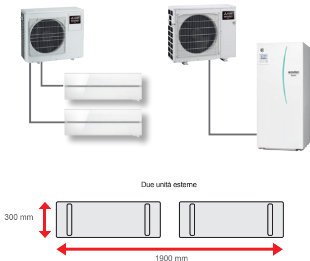
Climatizzatore aria/aria
