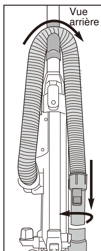
Passez le boyau au-dessus de l'anneau de retenue. Pressez l'extrémité lâche dans le port d'entrée du boyau et tournez-la dans le sens horaire pour la verrouiller en place.
