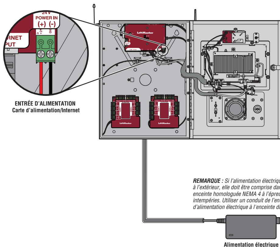
Alimentation électrique
