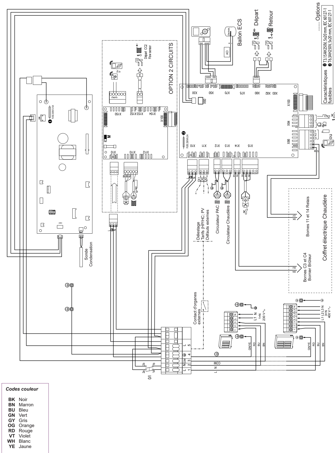
fig. 60 - Câblage électrique module hydraulique (PAC)
