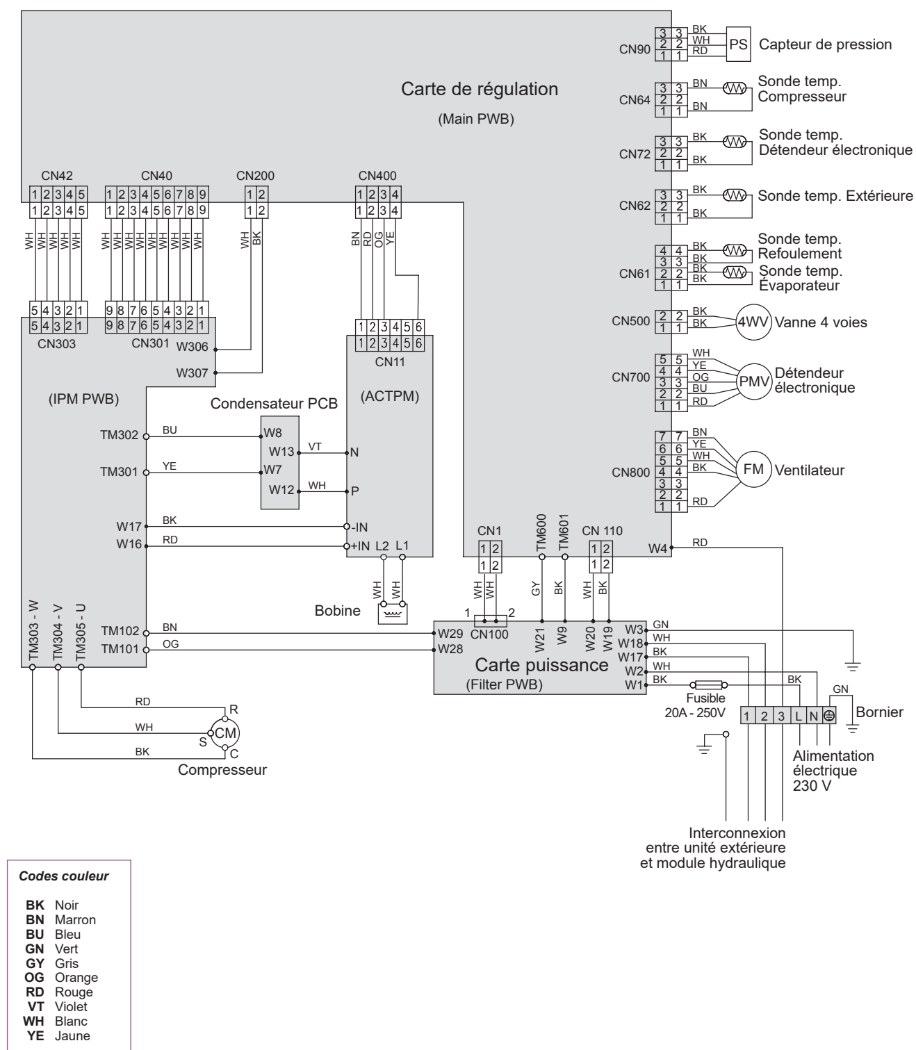
fig. 57 - Câblage électrique unité extérieure Alféa Hybrid Duo Fioul A.I. 8
