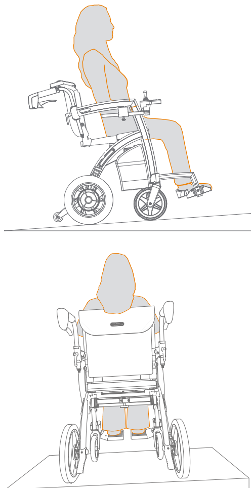
Figure 53: L'angle de pente maximal est de 6° / 10,5% (en haut) et l'angle latéral maximal est de 6° / 10,5% (en bas).
