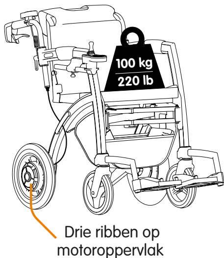
Figuur 1: Rollz Motion Electric en Rollz Motion Electric 2 breedte en maximale belasting.
