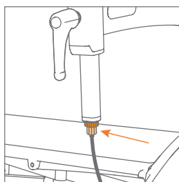
Abbildung 77: Bremseneinstellung über die Einstellschraube, direkt unter dem Sperring.
