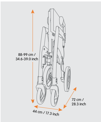
Figuur 82: Zo compact is de ingeklapte Rollz Motion Electric (2022). *46 cm / 18,1 inch voor het Rollz Motion Electric2 (2024) model.
