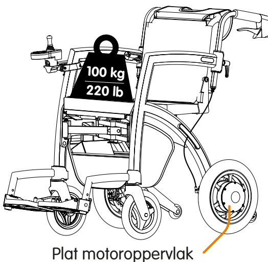
Figuur 1: Rollz Motion Electric en Rollz Motion Electric 2 breedte en maximale belasting.
