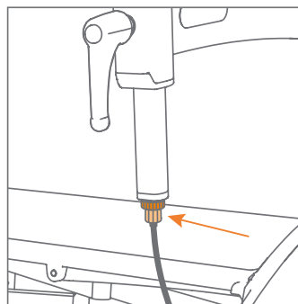
Figuur 77: Remafstelling via de afstelmoer, net onder de vergrendelingsring.
