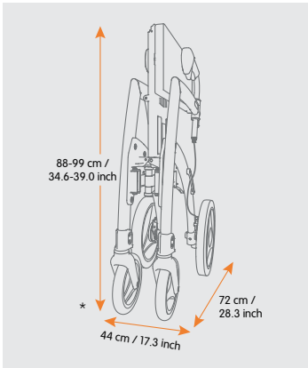
Abbildung 82: So kompakt ist der zusammengeklappte Rollz Motion Electric (2022). *46 cm / 18,1 Zoll für der Rollz Motion Electric 2 (2024) Modell.
