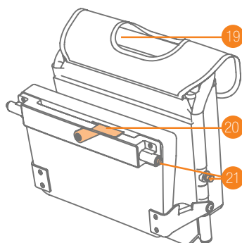
Figuur 4: Rolstoelpakket.
