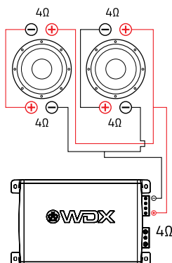
2 X 4Ω DVC SUBWOOFER
