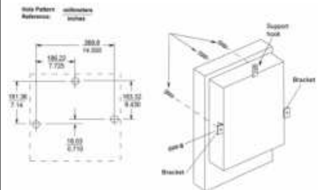
Figure 4 : Montage sur une surface, panneau ou mur (vue arrière)
