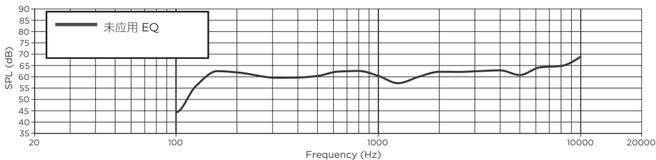
轴上频率响应
