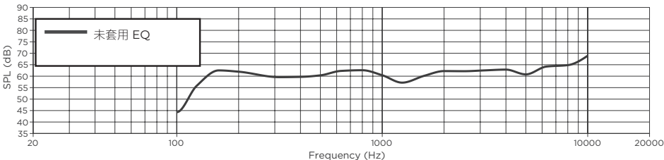
軸線上頻率響應
