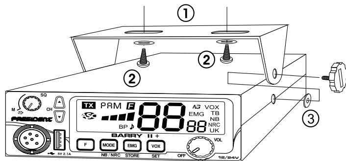
Schemat montażu
