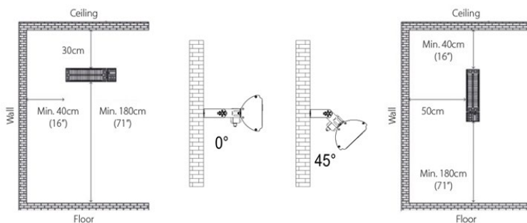
Diagrama 1: Montado en la pared, horizontal o vertical
