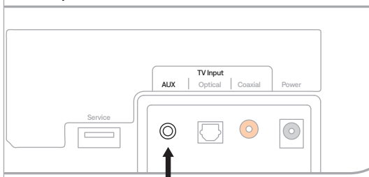
Panel de puertos de la barra de sonido
