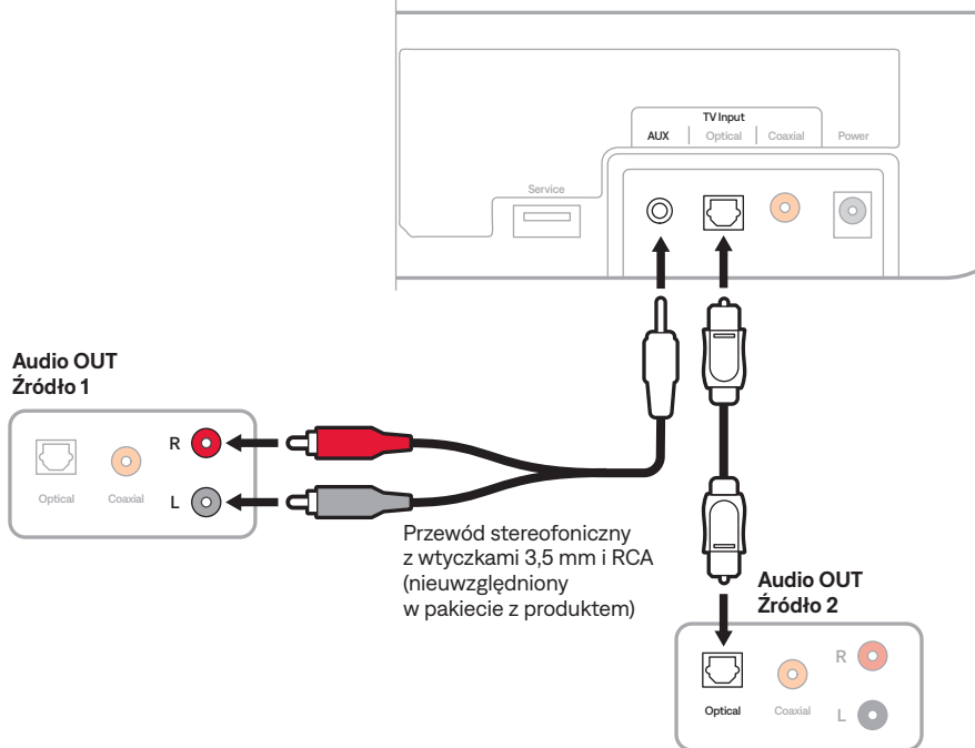
Złącza listwy dźwiękowej
