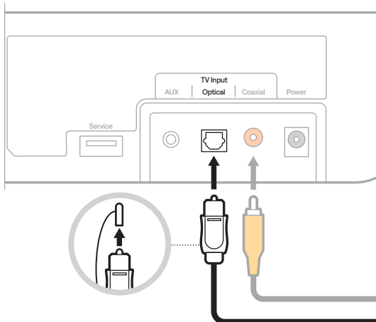
Panel de puertos de la barra de sonido
