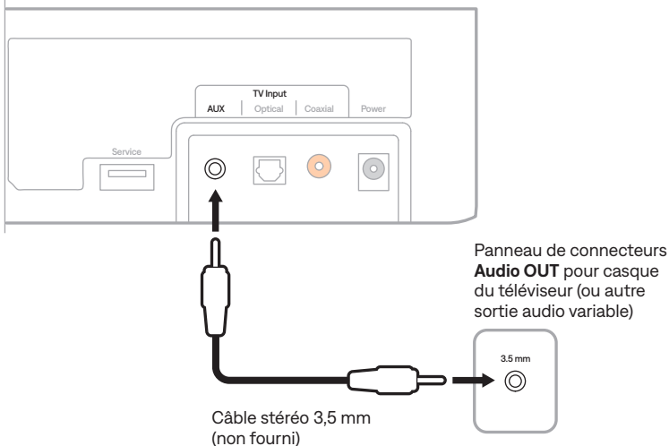
Panneau de connecteurs de la barre de son
