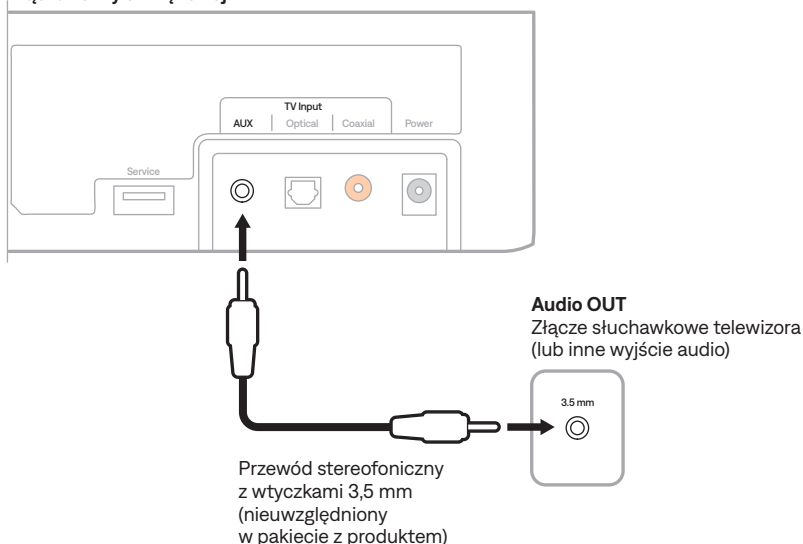
Złącza listwy dźwiękowej
