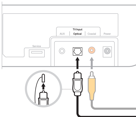
Pannello porte della soundbar
