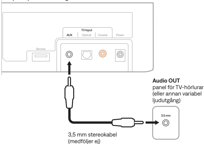
Portpanel på soundbarhögtalare
