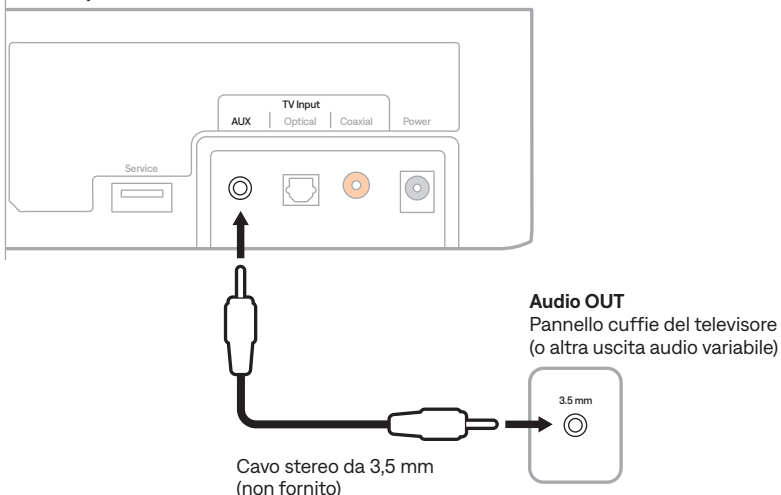
Pannello porte della soundbar
