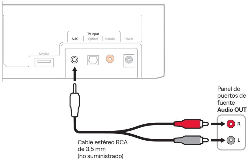
Panel de puertos de la barra de sonido
