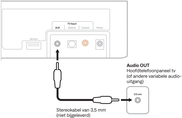
Aansluitpaneel soundbar
