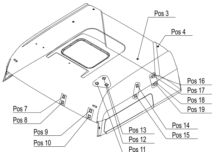
Fig. 38a: XXL-Fhs (L/R45) ESC-506a
