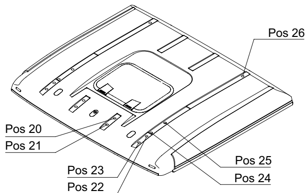
Fig. 38d: XL; L und M-Fhs (L/R 44; 34; 17) ESC-506d
