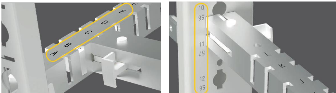
Figure 4 - Les repères sur les traverses garantissent un montage sans erreur
