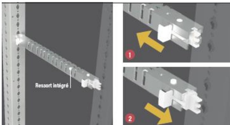
Figure 3 - Fixation des traverses grâce à des inserts à ressort
