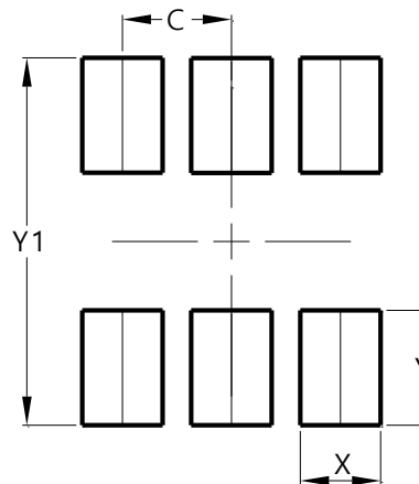
TSOT26 (Standard)
