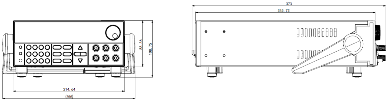
详细尺寸图
