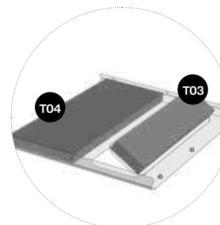
Einkleben des Schallschutzes T03 n der unteren Kante der Lamelle T04 mittig
