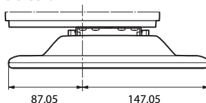
Derecha mm
