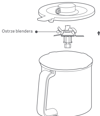
Zaczep ostrza blendera
