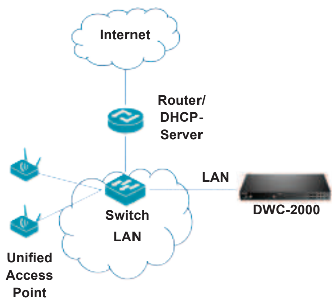
Abbildung 10. Netzwerktopologie
