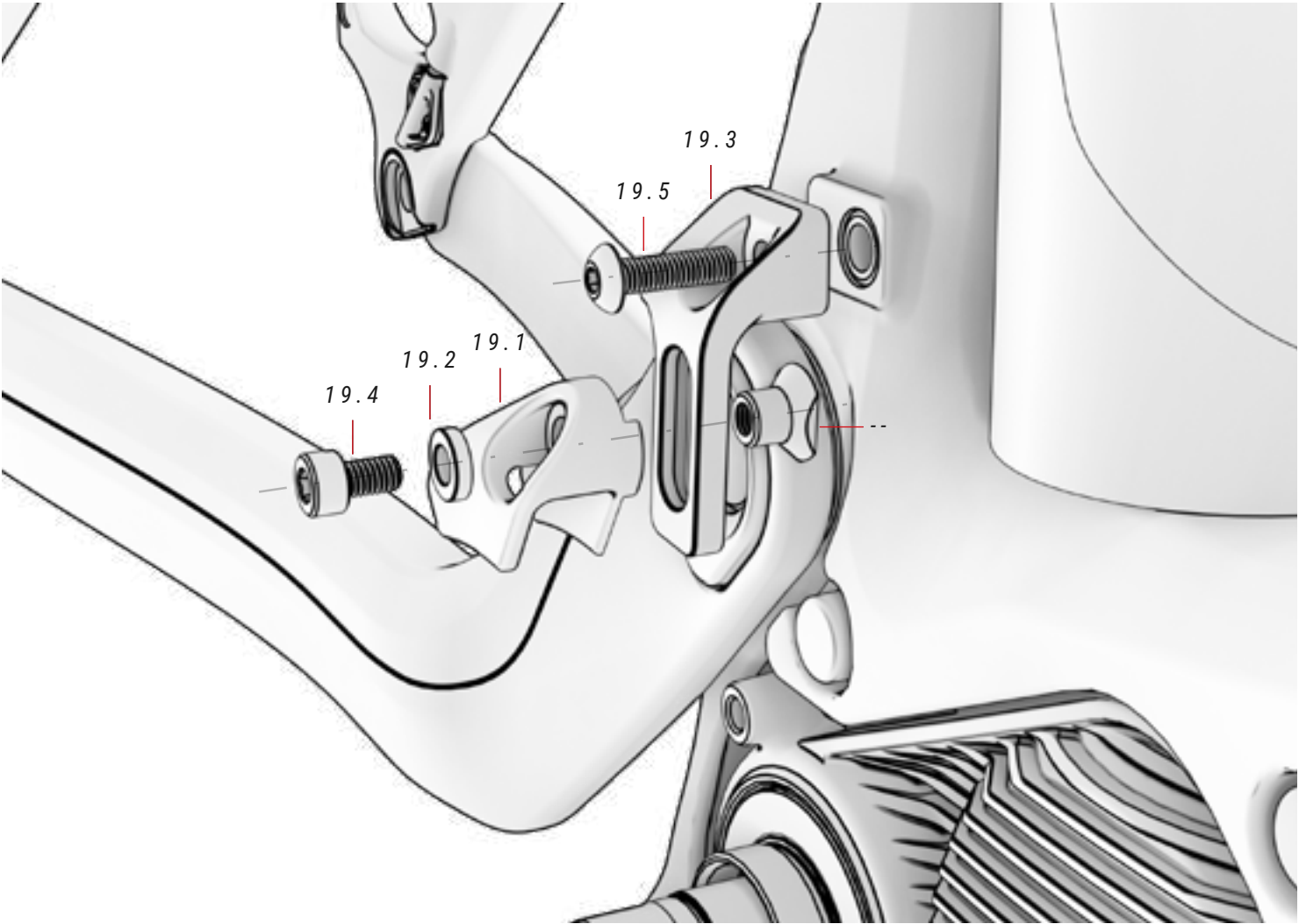
19 CHAINGUIDE ref.: 363300900
