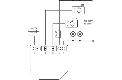
Fig. 1: Esquema eléctrico básico
