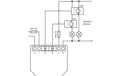
Abb. 1: Basis-Anschlussplan
