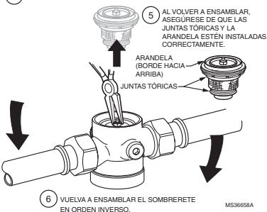
Fig. 4. Remplazar el cartucho FK06.
