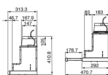
側視圖
