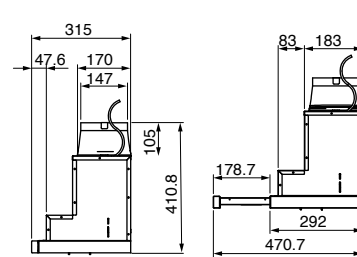
側視圖
