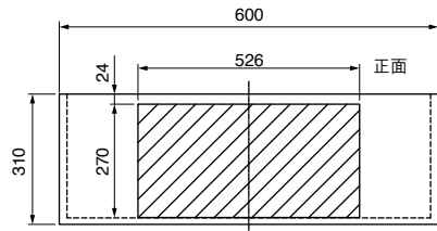
底視圖
