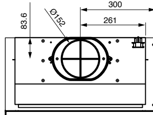
頂視圖
