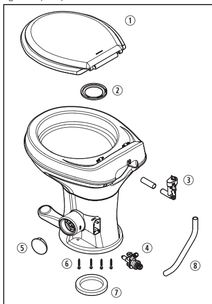
13 Pièces détachées de la série 300
