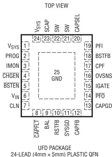
LTC4041EUFD LTC4041IUFD
