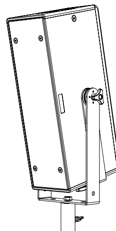
STÄNDERINSTALLATION
