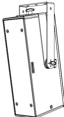
HÄNGEINSTALLATION AN GITTERTRÄGER
