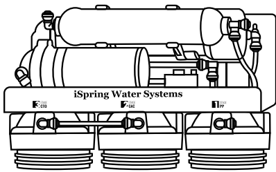
RO-Maschinenkopf (Membran noch nicht installiert)
