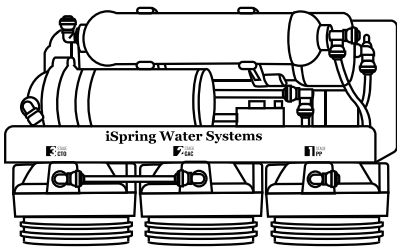
Tête de la machine d'OI (la membrane n'est pas encore installée)
