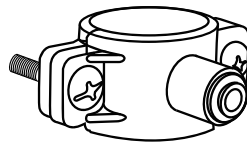
Raccordo di scarico da 1/4" (0,635 cm) (articolo nr. ADS1K)
