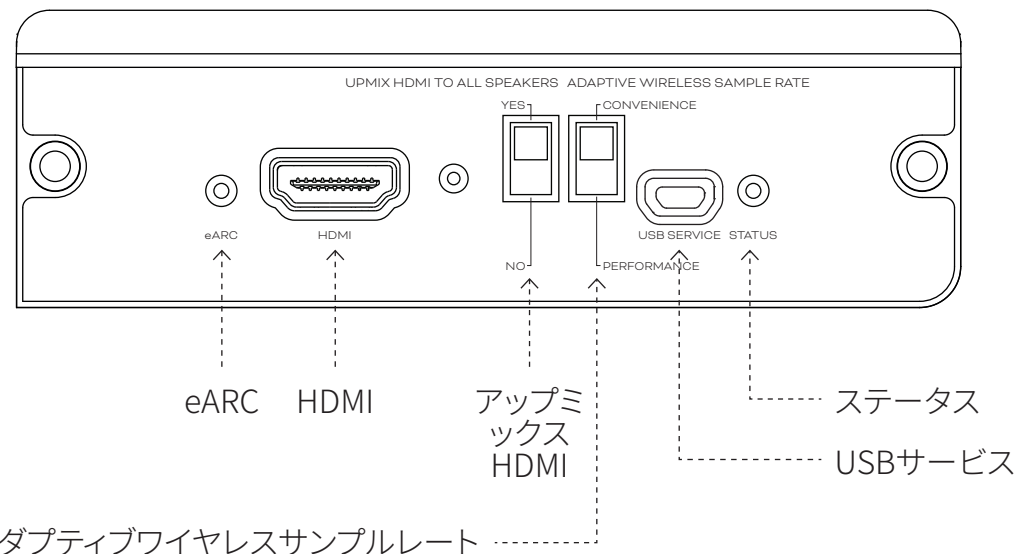
D 10:HDMIモジュールの背面パネル
