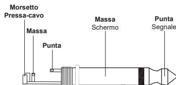
Uso Sbilanciato del connettore jack da 6.3mm TS
