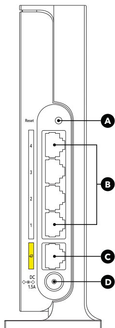
Illustration 3 : Panneau arrière.
