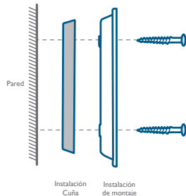
Con cuña de montaje de 15°
