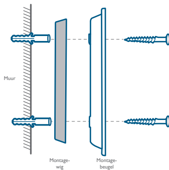
Met montage-gewig van 15°
