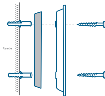
Com a cunha de instalação de 15°
