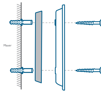
Mit 15°-Montagekeil
