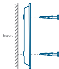
Montage de mural Sans cale de montage 15°
