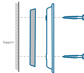
Montage de Cale Montage de mural Avec cale de montage 15°
