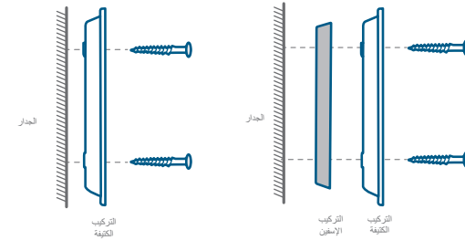
بدون إسفين متصاعد بمقدار 15 درجة
