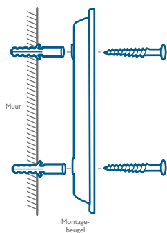
Zonder montage-gewig van 15°
