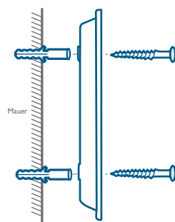
Ohne 15°-Montagekeil
