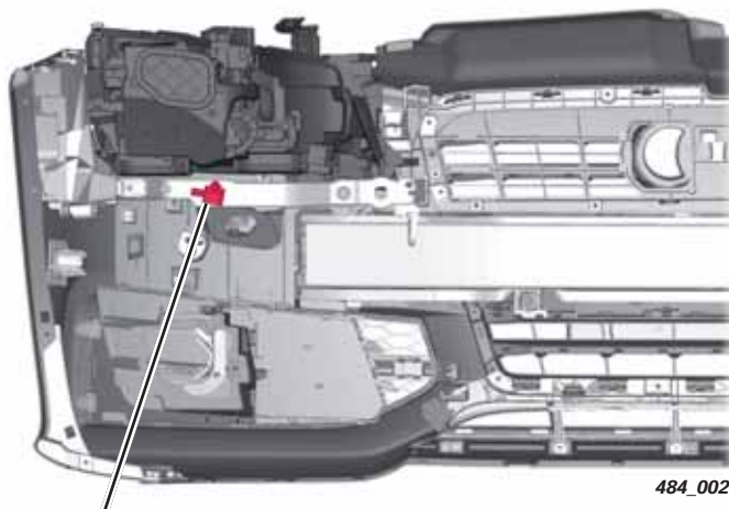
Crash sensor G283
