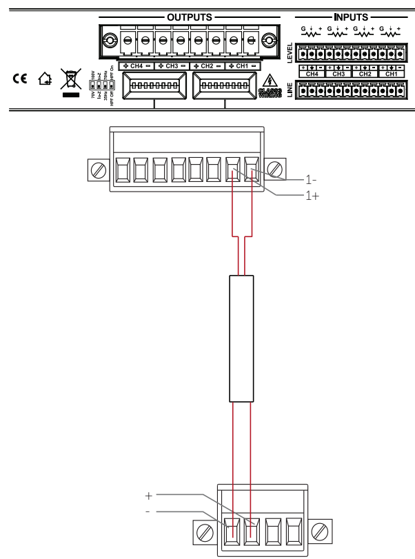
Figure 4.4: Bias Q1/Q2
