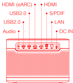
Vue arrière
