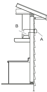
A. Bouche de décharge sur le mur B. Conduit rond de 6" (15,2 cm)
