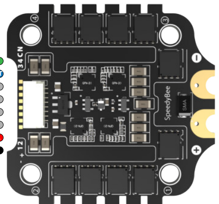
BLS 50A 4-in-1 ESC
