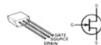
2SK192A GR Q15, Q17, Q19, Q21, Q29
