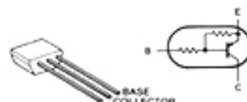
RN2202 Q10
