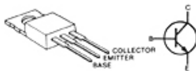
2SC1971 Q1
