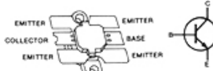
2SC2904 Q5, Q6
