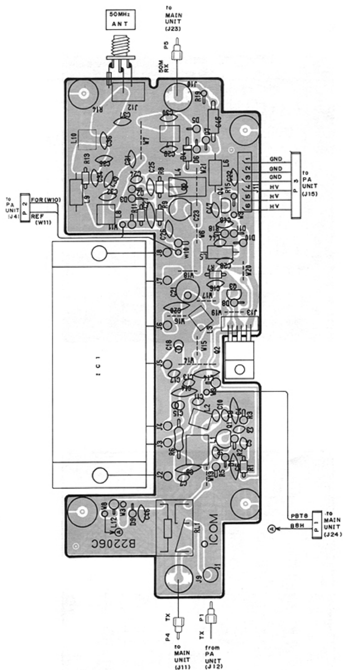
2SC2407(A) Q1
