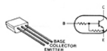
RN1202 Q25, Q35, Q44
