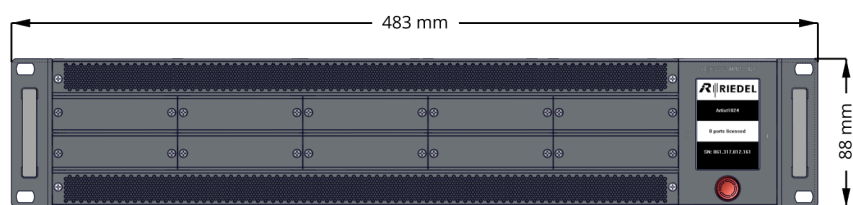
图 13 : Artist-1024 寸法图 (正面图)
