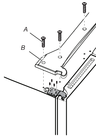
A. Vis du couvre-charnière supérieur
