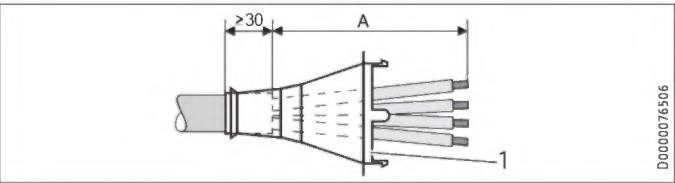
1 Кабельная втулка
